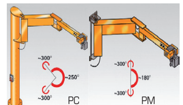
Construction 8: à bras articulée
